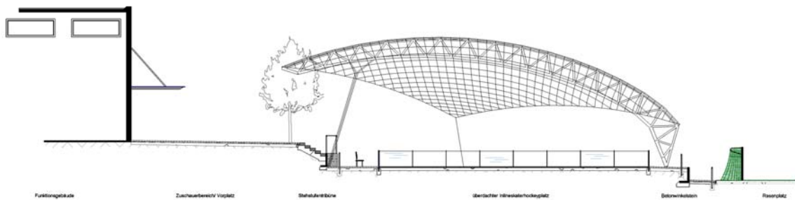
Multifunktionsfläche mit Membrandach
