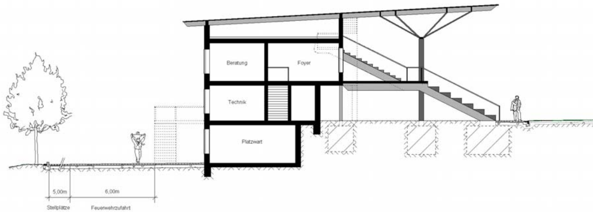
Westtribüne mit Funktionsgebäude
